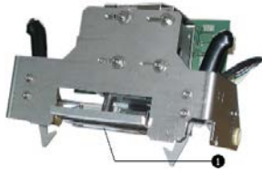
Fig. 54: Thermal printer
