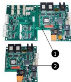
Fig. 67: PCB MC Barcode Mainboard
