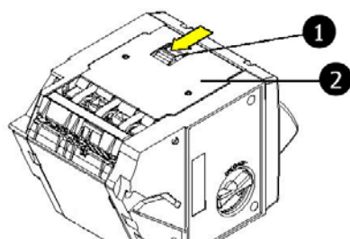
Fig. 98: Apertura della cassetta rendiresto
