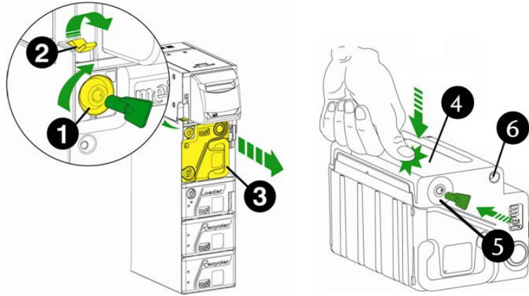
Fig. 102: Estrazione e apertura della cassetta terminale
