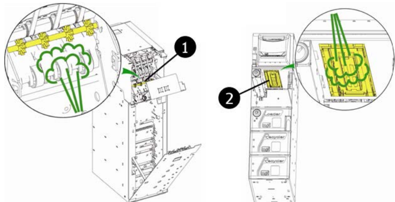
Fig. 112: Pulizia dal basso dell'unità di controllo e del modulo principale
