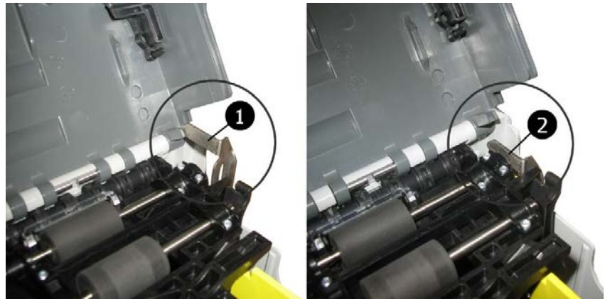
Fig. 104: Cassetta di caricamento, sistema di bloccaggio posizione corretta (sinistra), posizione errata (destra)
