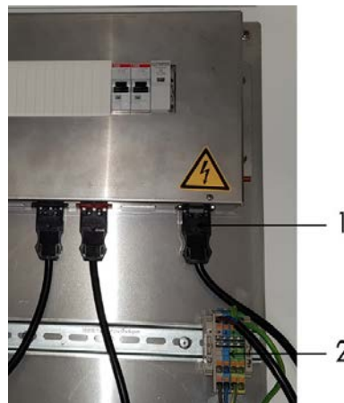
Fig. 21: Morsettiera -X0
