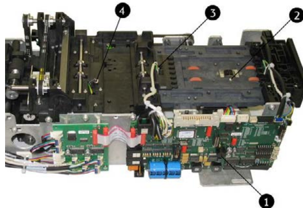
Fig. 61: LED Live e barriere fotoelettriche per l'analisi degli errori
