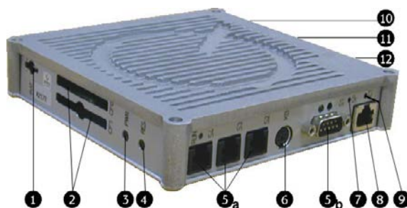
Fig. 41: TCC (Tipo LCC)
