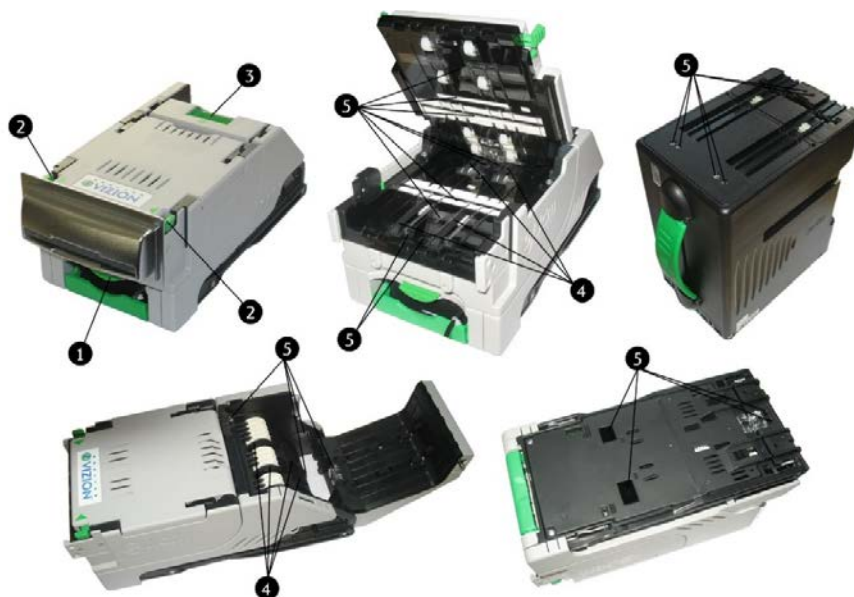
Fig. 83: Pulizia dell'unità NBA
