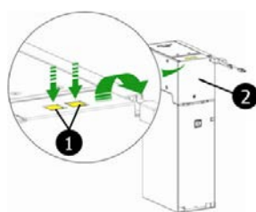
Fig. 107: Apertura della copertura dell'unità di controllo
