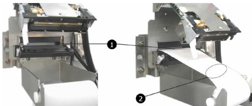
Fig. 74: Inserimento della carta nel dispositivo di avanzamento
