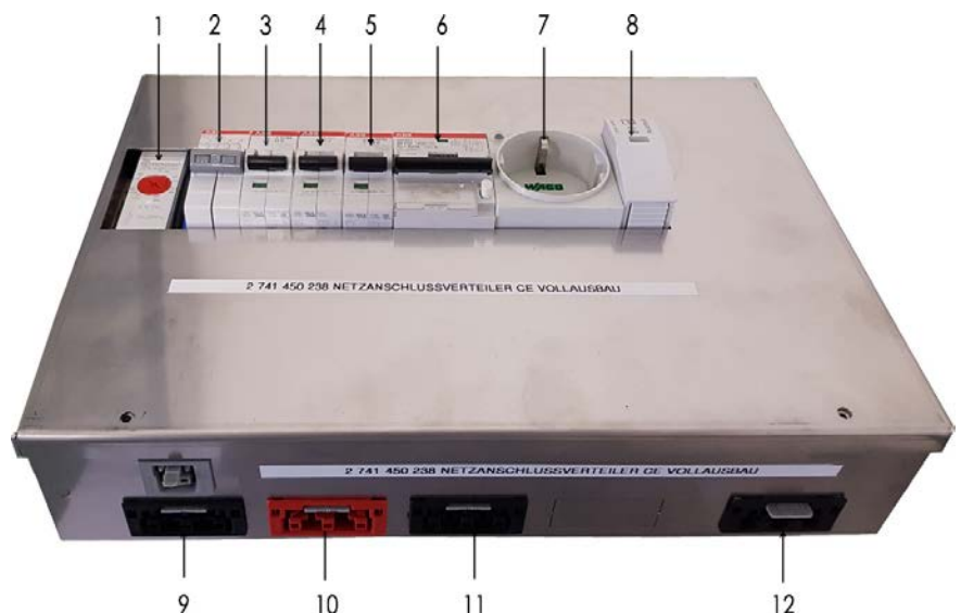
Fig. 15: Pannello di alimentazione (figura con opzioni)
