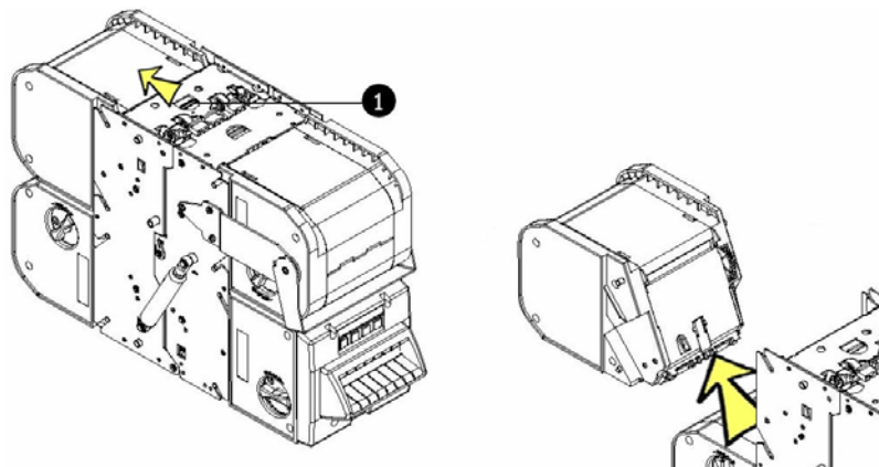
Fig. 95: Estrazione delle cassette di ricircolo o della cassetta (Multi-)Escrow
