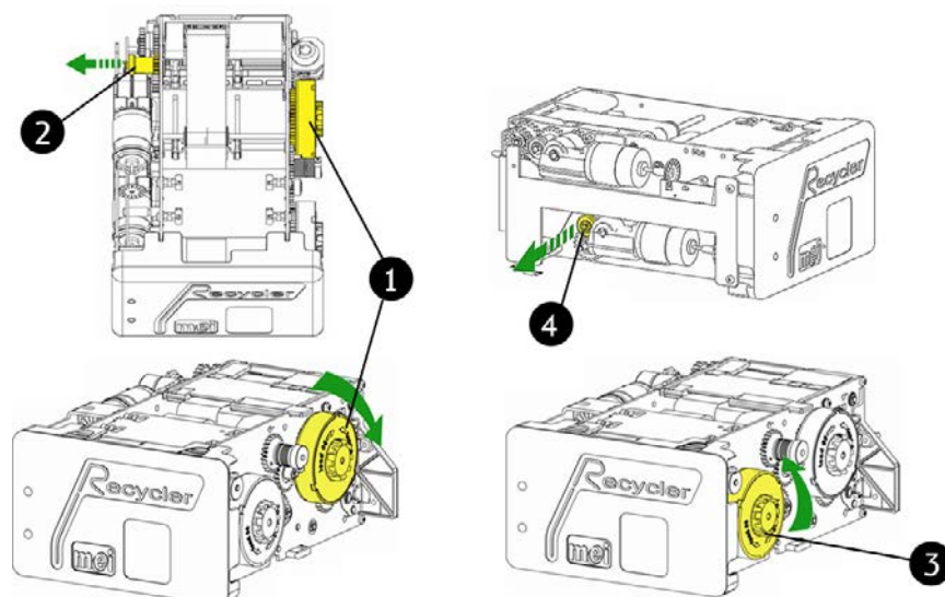
Fig. 116: Cassette di ricircolo: rimozione di un blocco di banconote
