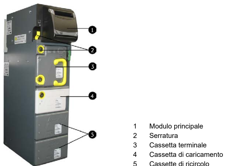
Fig. 100: Riciclatore di banconote BNR MEI
