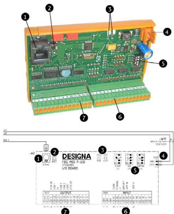
Fig. 45: Scheda I/O- "Midi-P-USI" (qui configurazione interfaccia I/O di un terminale di controllo ingressi)
