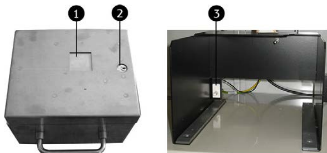
Fig. 79: Prelievo e apertura della cassetta delle monete
