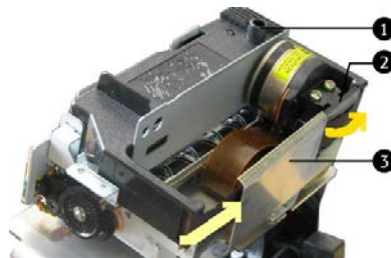
Fig. 60: Inserimento della cassetta nastro inchiostro
