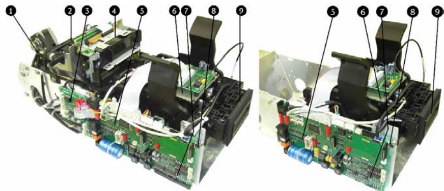
Fig. 47: Multicon nel sistema a banda magnetica (esempi di ampliamento per i terminali ENT (sx.) ed EXT (dx.))
