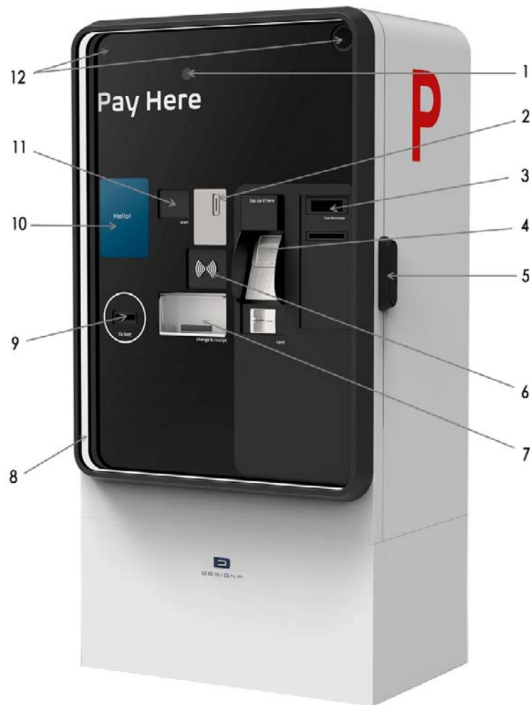
Fig. 7: Elementi di comando sullo sportello (figura con opzioni)
