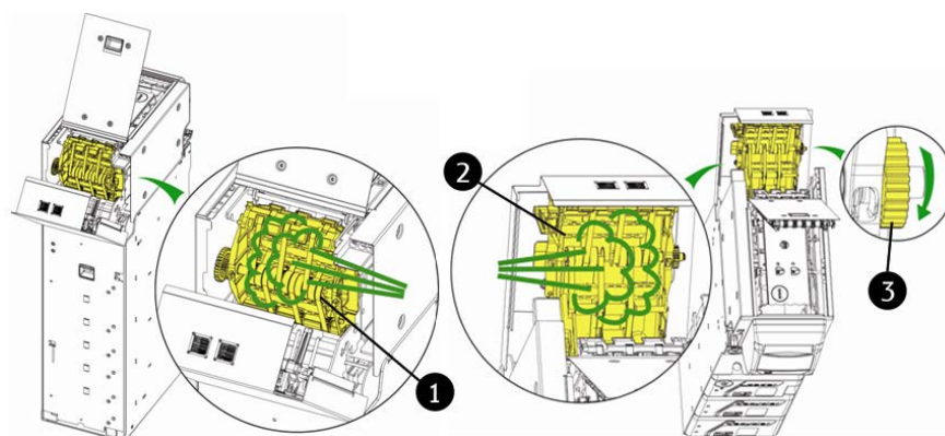
Fig. 110: Pulizia dell'unità di controllo
