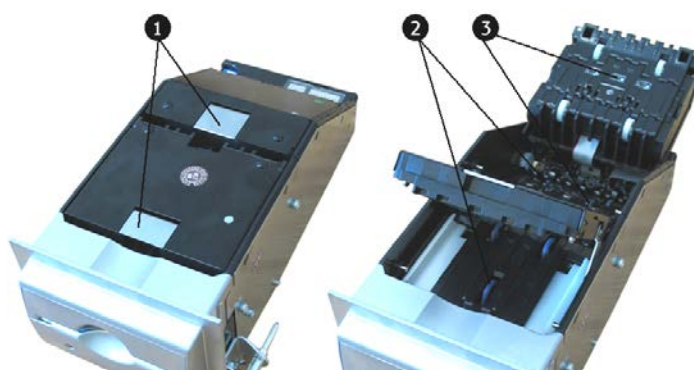
Fig. 90: Pulizia del lettore di banconote
