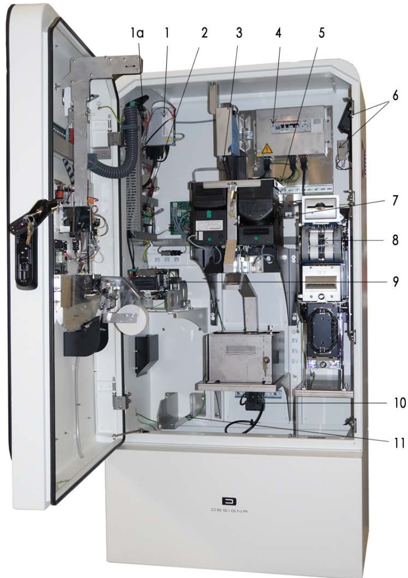
Fig. 10: Componenti all'interno del terminale (figura con opzioni)
