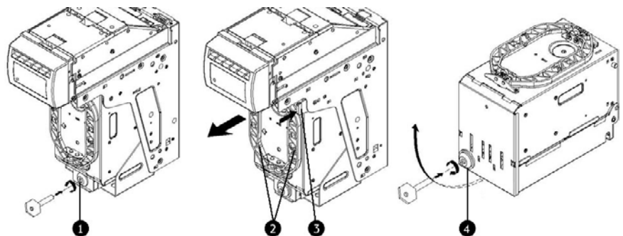
Fig. 85: Estrazione e apertura della cassetta (figura con opzioni)
