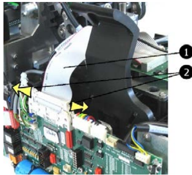
Fig. 59: Sgancio del cavo a nastro piatto
