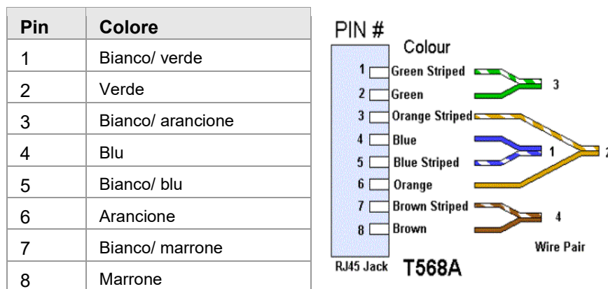
Fig. 35: Assegnazione presa Ethernet, EIA/TIA-T568A
