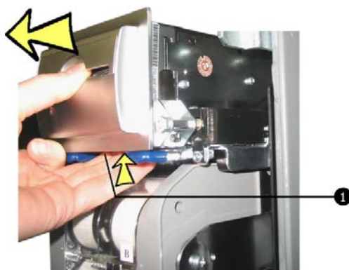
Fig. 89: Estrazione del lettore di banconote
