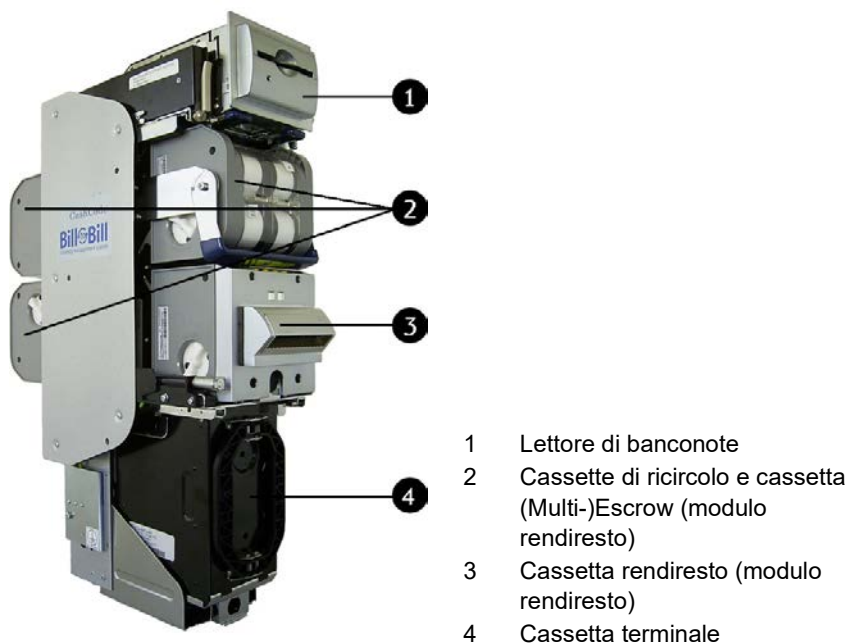
Fig. 87: Ricircolatore di banconote BNR CASHCODE
