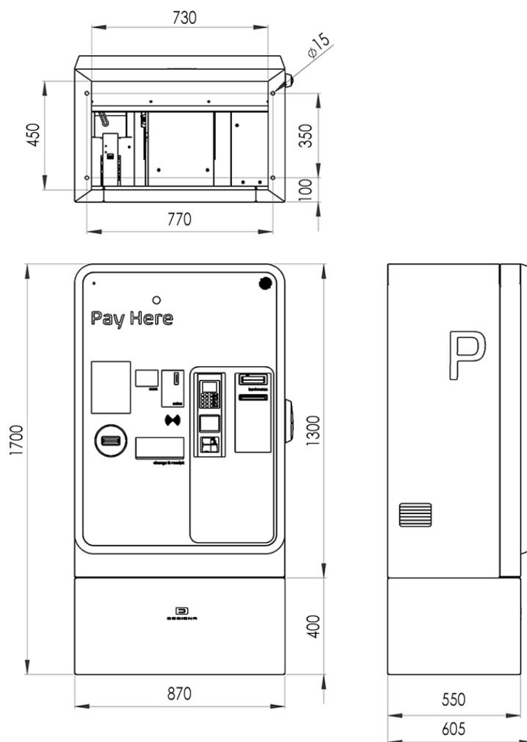
Fig. 5: Pay Cash&Card, con cornice luminosa opzionale, dimensioni in mm
