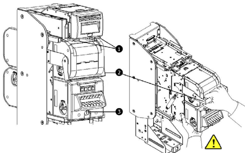
Fig. 91: Prelievo del modulo rendiresto
