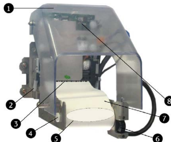
Fig. 71: Stampante delle ricevute
