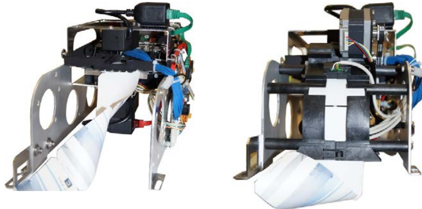
Fig. 69: Multicon MC Barcode: senza doppia unità di alimentazione (sinistra), con doppia unità di alimentazione (destra)
