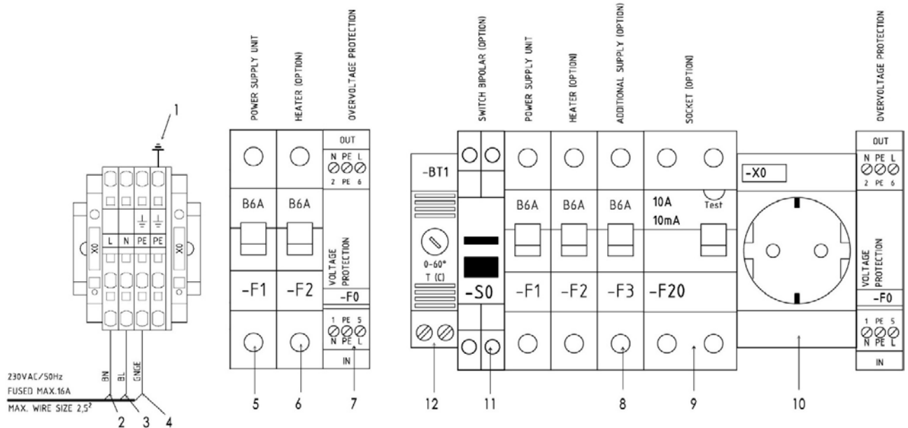
Fig. 32: Morsettiere -X0, pannello di alimentazione (equipaggiamento di base e equipaggiamento con opzioni)
