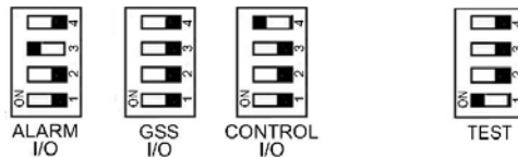
Fig. 46: Posizioni DIP-switch
