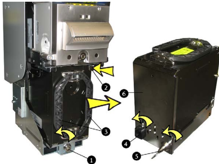
Fig. 88: Prelievo e apertura della cassetta terminale
