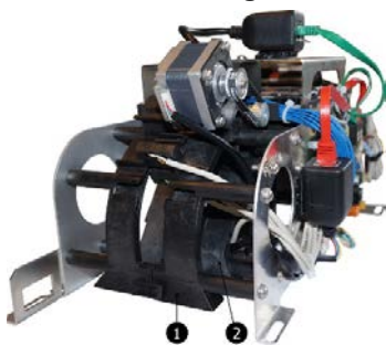
Fig. 63: Doppia unità di alimentazione (opzione)
