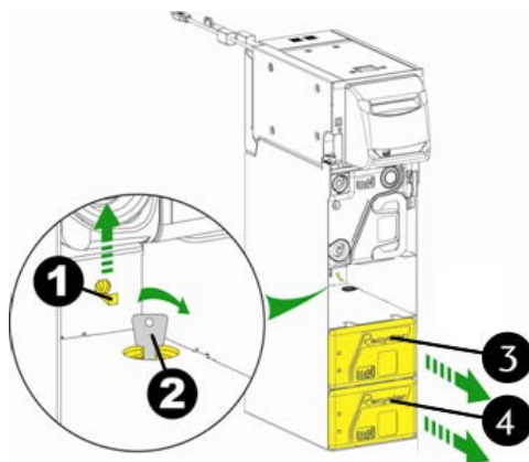
Fig. 115: Estrazione della cassetta di ricircolo
