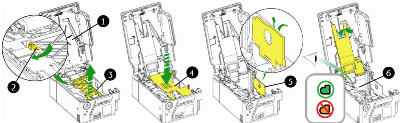
Fig. 106: Inserimento delle banconote
