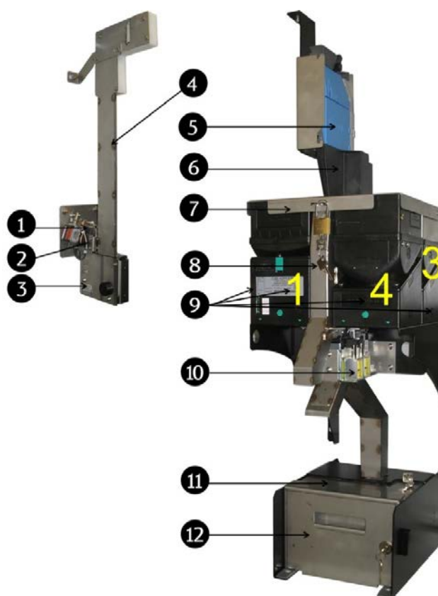
Fig. 76: MVE; sullo sportello (a sinistra), all'interno del terminale (a destra)
