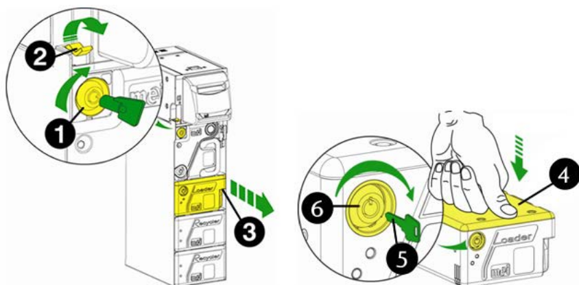
Fig. 103: Estrazione e apertura della cassetta di caricamento
