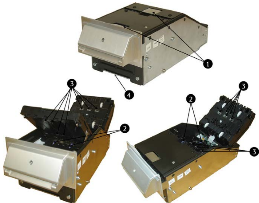
Fig. 86: Pulizia dell'unità MFL
