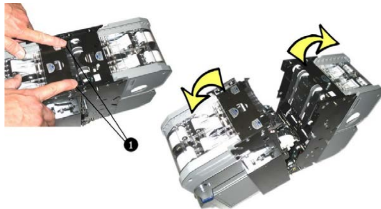
Fig. 92: Apertura del modulo rendiresto
