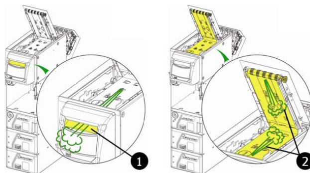
Fig. 109: Pulizia della fessura di accettazione delle banconote e dell'unità di posizionamento
