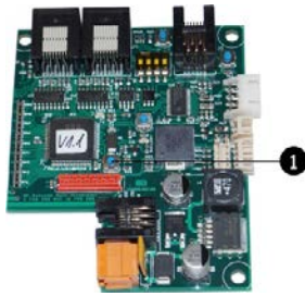
Fig. 62: Reset button
