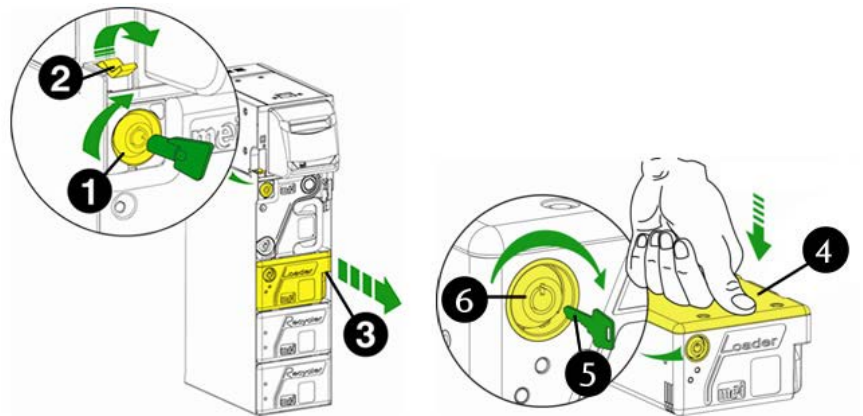
Abb. 92: Ladekassette entnehmen und öffnen
