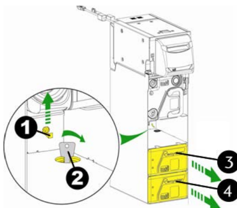
Abb. 104: Recycling-Kassette entnehmen
