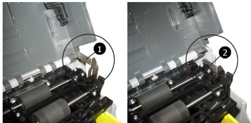
Abb. 93: Ladekassette, Verschluss-Riegel: richtige Position (links), falsche Position (rechts)
