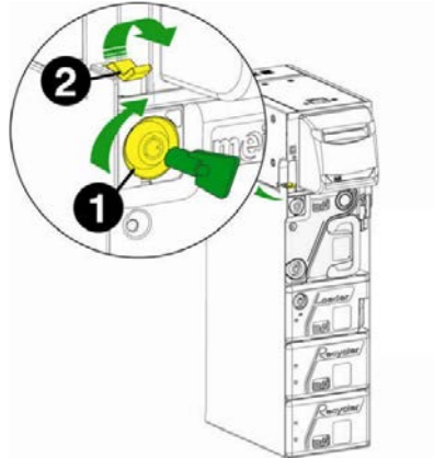
Abb. 90: Verriegelung
