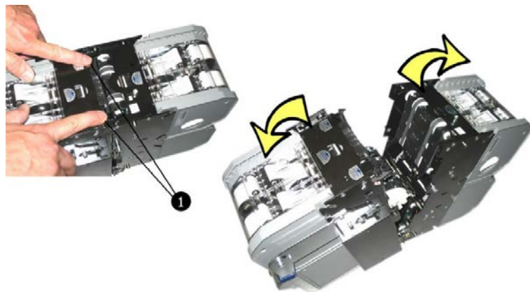
Abb. 81: Wechsel-Modul öffnen
