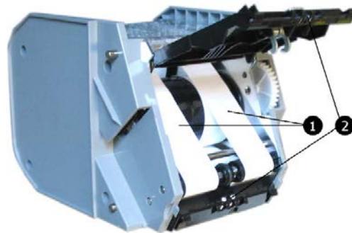
Abb. 86: Recycling- oder (Multi-)Escrow-Kassette reinigen
