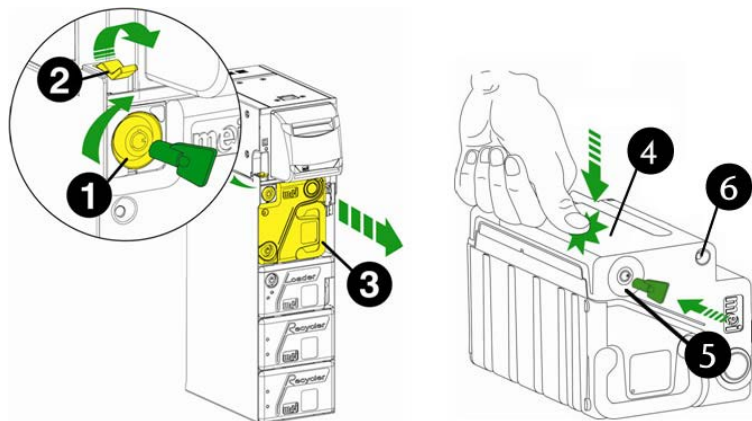
Abb. 91: Endkassette entnehmen und öffnen
