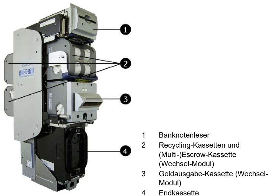
Abb. 76: Banknoten-Recycler BNR CASHCODE
