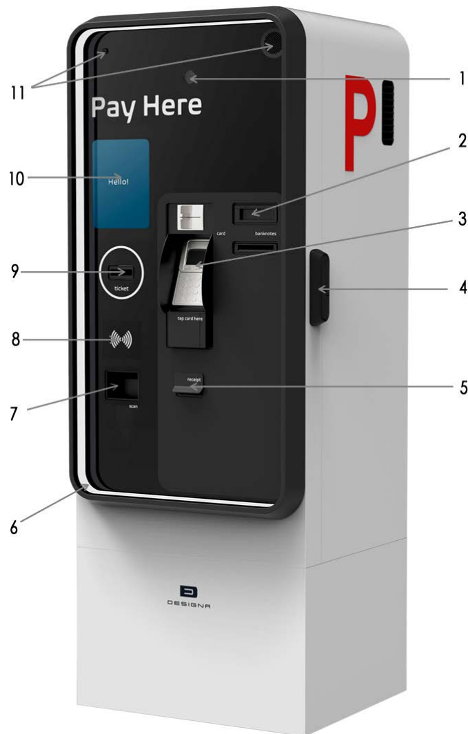
Abb. 7: Bedienelemente an der Tür (Abbildung mit Optionen)
