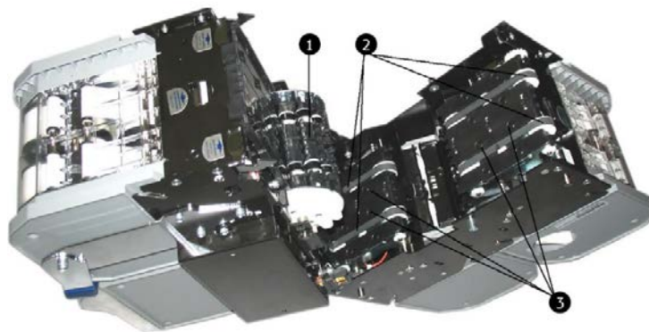
Abb. 82: Wechsel-Modul reinigen
