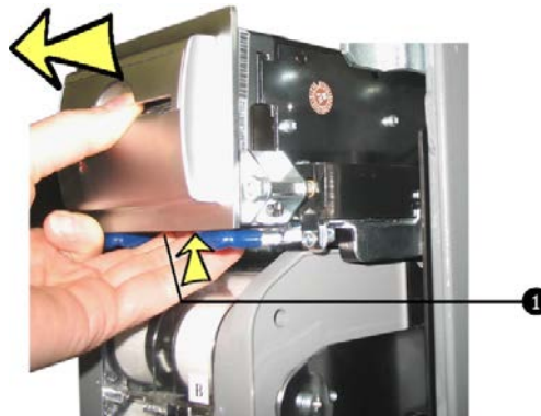
Abb. 78: Banknotenleser entnehmen
