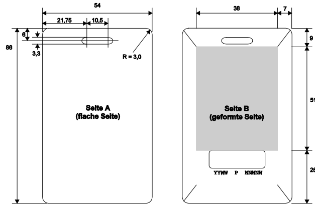
Abb. 107: Maße in mm: EasyMove-Karte
