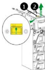
Abb. 97: Positionierer-Abdeckung öffnen
