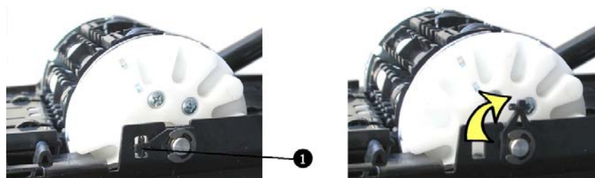
Abb. 83: Transportweg-Schalter entnehmen
