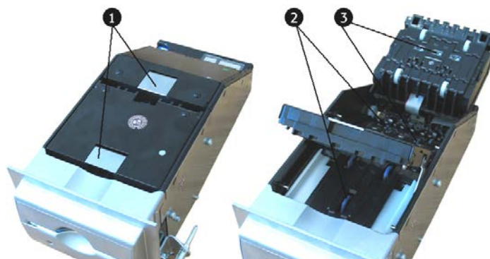
Abb. 79: Banknotenleser reinigen
