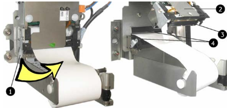
Abb. 75: Öffnungshebel lösen und Druckereinheit von der Papierrolle lösen
