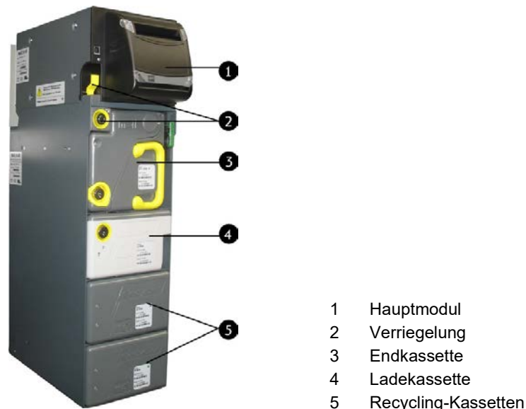
Abb. 89: Banknoten-Recycler BNR MEI
