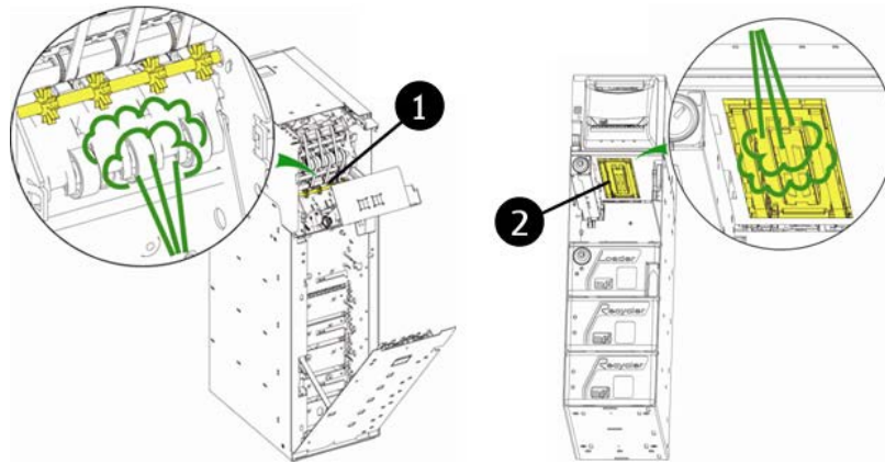
Abb. 101: Prüfeinheit und Hauptmodul von unten reinigen
