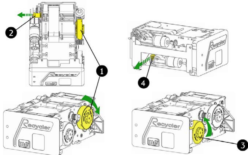
Abb. 105: Recycling-Kassette: Banknotenstau beseitigen
