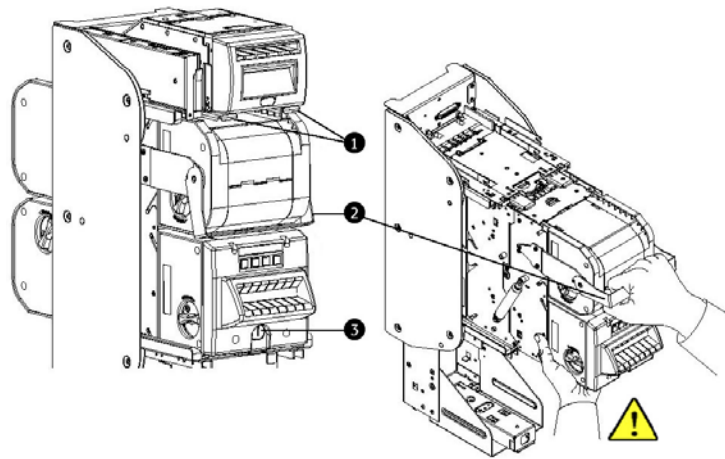
Abb. 80: Wechsel-Modul entnehmen
