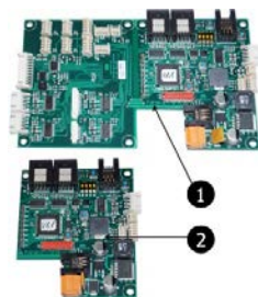
Abb. 66: FBG MC Barcode Mainboard
