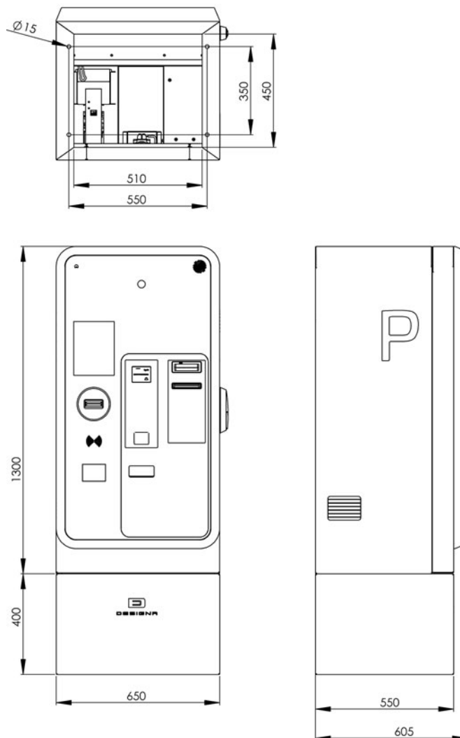
Abb. 5: Pay Coinless, mit optionalem Leuchtrahmen, Abmessungen in mm
