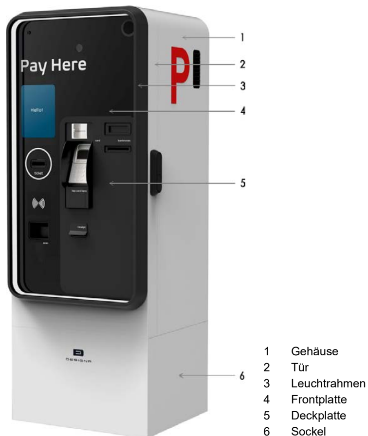
Abb. 6: Allgemeiner Aufbau (Abbildung mit Optionen)
