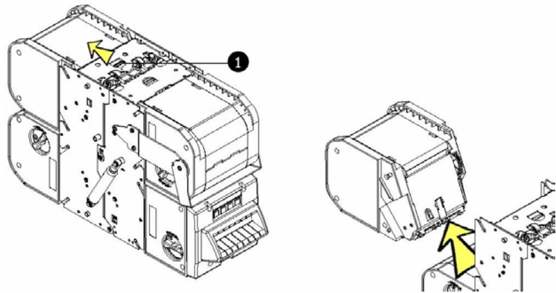
Abb. 84: Recycling- oder (Multi-)Escrow-Kassette entnehmen
