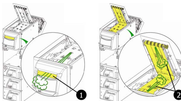
Abb. 98: Banknoten-Annahme und Positionierer reinigen
