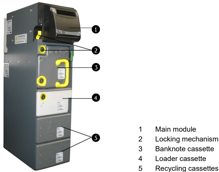
Fig. 90: Banknote recycler BNR MEI
