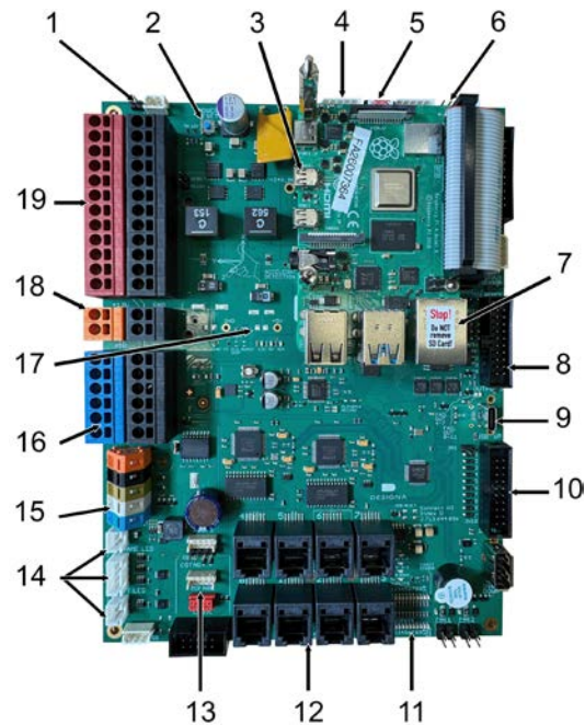
Abb. 28: SBC Mainboard V3
