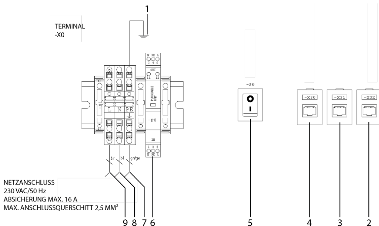
Abb. 19: Klemmleiste -X0, Netzanschlussverteiler
