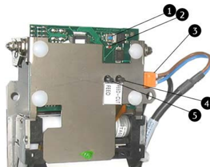
Abb. 32: FBG Quittungsdrucker
