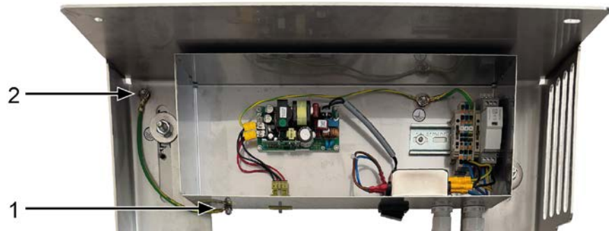
Abb. 24: Messpunkte
