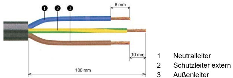
Abb. 20: Netzzuleitung abisolieren
