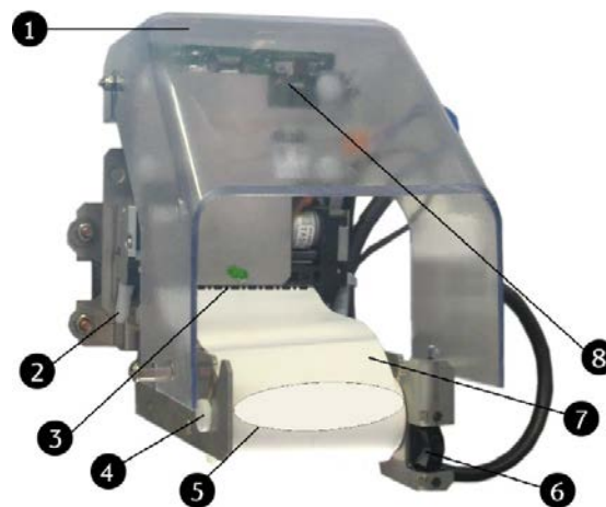
Abb. 30: Quittungsdrucker (Abbildung ähnlich)
