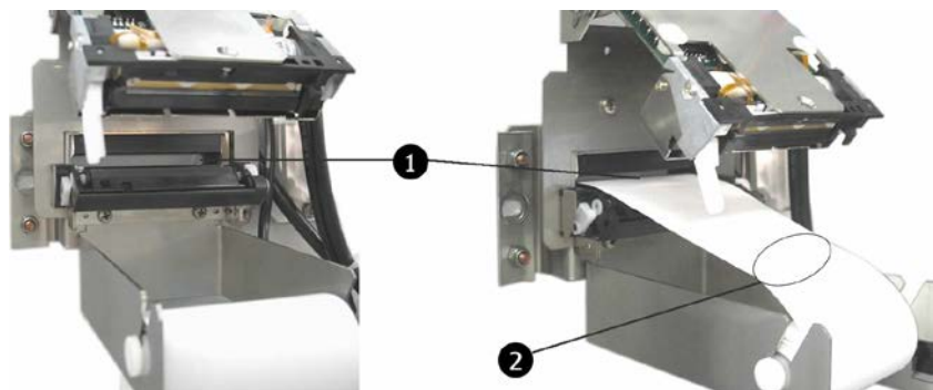
Abb. 33: Papier in Einzug fädeln
