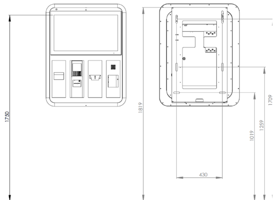
Abb. 15: Montagehöhe
